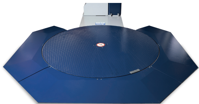
OPTIONAL RAMPA 270° OPTIONAL 270° RAMP Optional rampa completa, per carico/scarico 270°, ideale per transpallet manuale. Optional complete ramp, for 270° loading/unloading, ideal for hand pallet truck.
